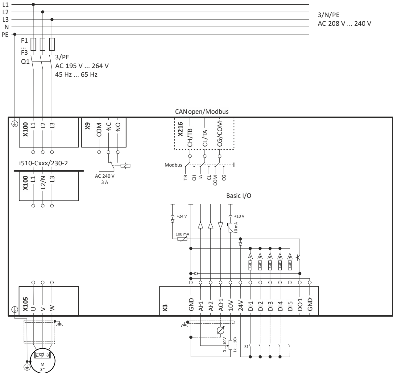
Fig. 4: Wiring example
